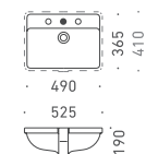
6 洗面器・手洗器 STARCK3 FAA70-2217 W490×D365 (ボウル内寸法) 4.5L ホワイト / 陶器 オーバーフロー付き 水栓穴：●＝穴あき ○＝穴あけ可 対応排水金具：A
