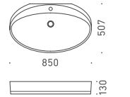
3-5 洗面器 ASN70-0002 W850×D507 22L ホワイト / 陶器 オーバーフローなし 水栓穴: ○ = 穴あけ可 対応排水金具: B
