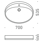
1,2 洗面器 ASN70-0001 W700×D535 9.2L ホワイト / 陶器 オーバーフローなし 水栓穴: ○ = 穴あけ可 対応排水金具: B
