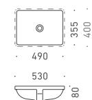
7 洗面器 STARCK3 FAA70-2218 W490×D355 (ボウル内寸法) 4.8L ホワイト / 陶器 オーバーフロー付き 対応排水金具：A
