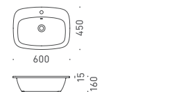
4 洗面器 GREEN ADF70-0303 W600×D450 3.8L ホワイト / 陶器 オーバーフロー付き 水栓穴：○＝穴あけ可 対応排水金具：A
