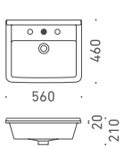
6 洗面器・手洗器 STARCK3 FAA70-2216 W560×D460 6.5L ホワイト / 陶器 オーバーフロー付き 水栓穴：●＝穴あき ○＝穴あけ可 対応排水金具：A
