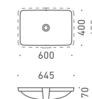
9 洗面器 LAUFEN PRO GAR70-0919 W600×D400 (ボウル内寸法) 10.5L ホワイト / 陶器 オーバーフロー付き 対応排水金具：A
