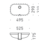
10 洗面器 D-CODE FAA70-3108 W495×D290 (ボウル内寸法) 7L ホワイト / 陶器 オーバーフロー付き 対応排水金具：A
