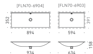
2,3 洗面器 SILENIO FLN70-6904 W894×D352 (ボウル内寸法) 7L FLN70-6903 W594×D352 (ボウル内寸法) 4L ホワイト / 銅板ホーロー オーバーフロー付き 対応排水金具：A
