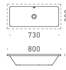
11 洗面器 NEW ZERO ADF70-3020 W730×D300 (ボウル内寸法) 6.5L ホワイト / 陶器 オーバーフロー付き 対応排水金具：A
