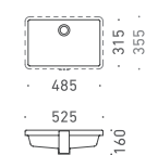
8 洗面器 VERO FAA70-0514 W485×D315 (ボウル内寸法) 7L ホワイト / 陶器 オーバーフロー付き 対応排水金具：A
