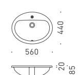
9 洗面器 LAUFEN PRO GAR70-0918 W560×D440 4.5L ホワイト / 陶器 オーバーフロー付き 水栓穴：●＝穴あき 対応排水金具：A
