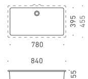
1 洗面器 CUBIC ALC70-0301 W780×D395 (ボウル内寸法) 14L ホワイト / 陶器 オーバーフロー付き 対応排水金具：A
