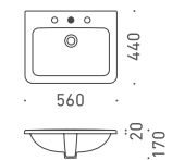
7 洗面器 LAUFEN PRO GAR70-0914 W560×D440 6.5L ホワイト / 陶器 オーバーフロー付き 水栓穴：●＝穴あき ○＝穴あけ可 対応排水金具：A
