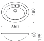
8 洗面器 DOLCEVITA ABA70-0006 W650×D480 4.5L ホワイト / 陶器 オーバーフロー付き 水栓穴：●＝穴あき ○＝穴あけ可 対応排水金具：A
