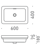
10 洗面器 CANOVA ROYAL ADF70-2310 W600×D400 9L ホワイト / 陶器 オーバーフロー付き 対応排水金具：A
